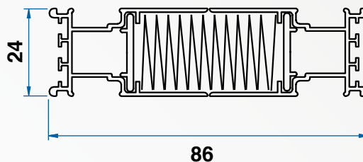
Profilo portarete
