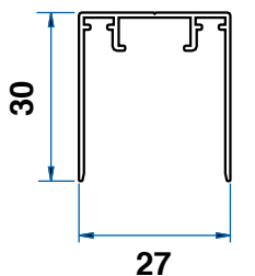
Guida superiore
