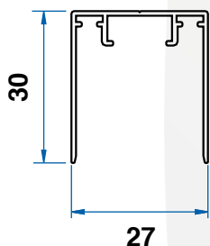
Guida superiore
