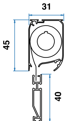
Cassonetto con tubo, rete e barra maniglia
